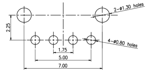
P.C.B Layout
